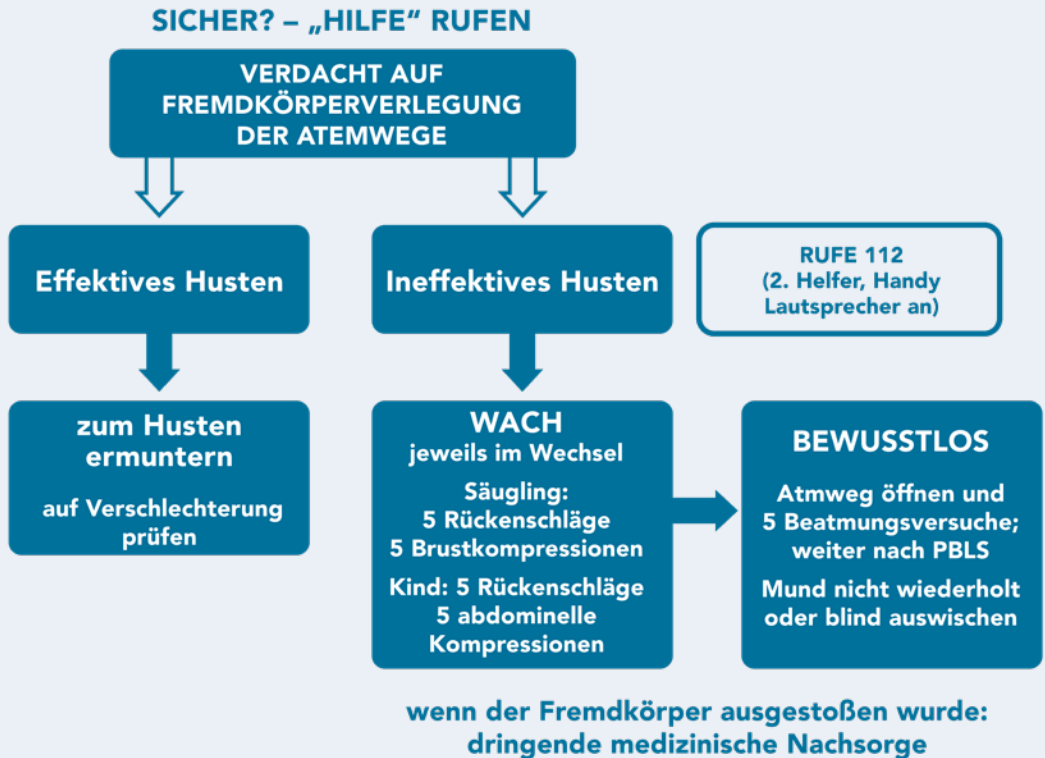
Abbildung 24 FBAO-Algorithmus
